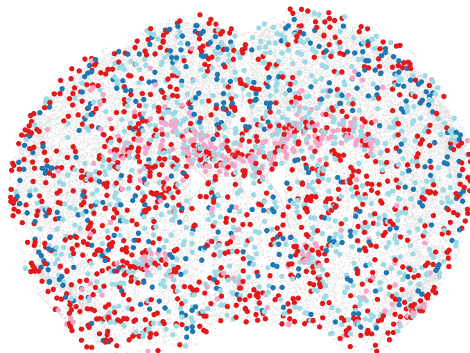
Popari
