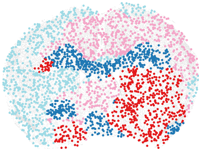
SpatialPCA
