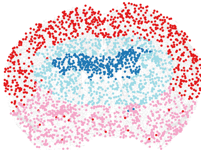
MEFISTO
